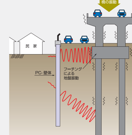
主な振動伝達パターン
