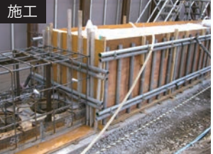
モルタル充填完了
