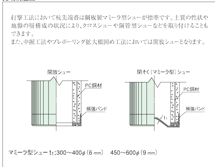
先端構造図
