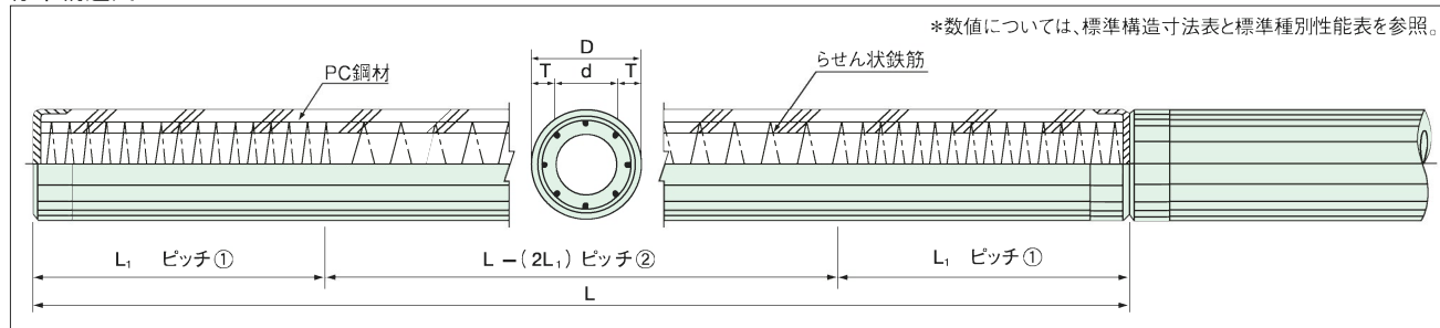
標準構造図
