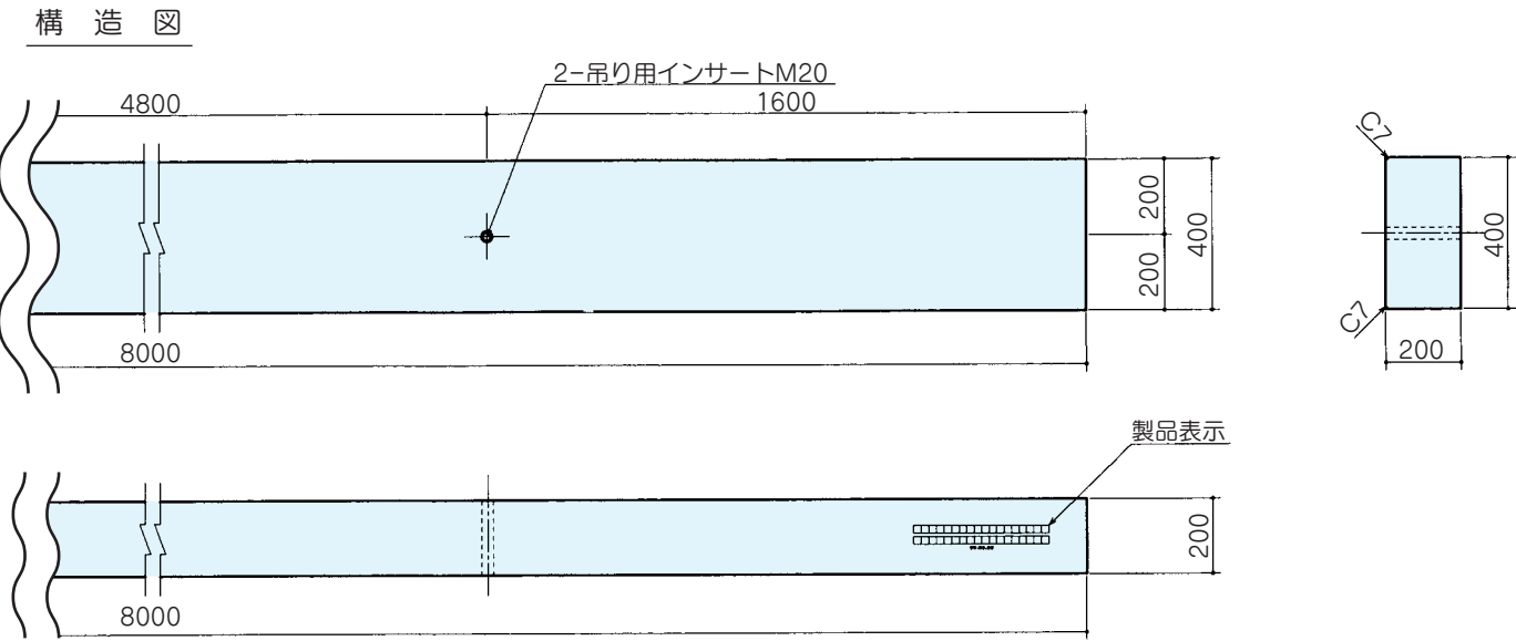
PCコンクリート板 構造図（8000×400×200）〔製品例〕
