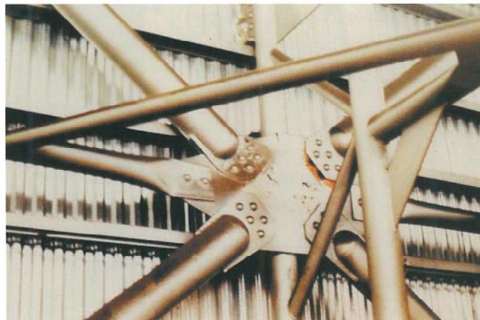
ブレース座屈とボルトの破断
