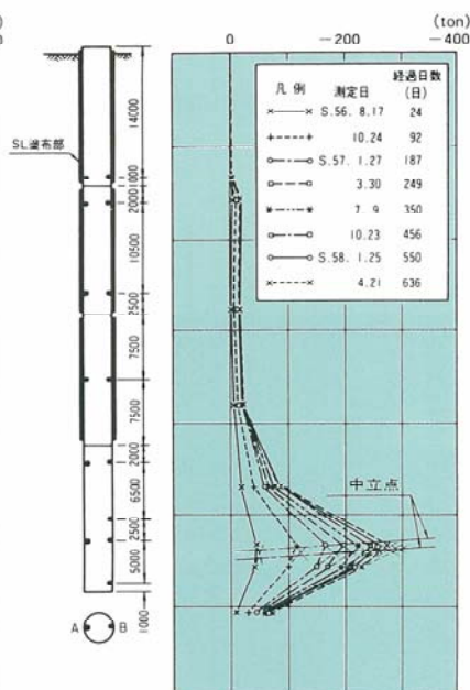
杭体軸力分布図 (SL杭)
