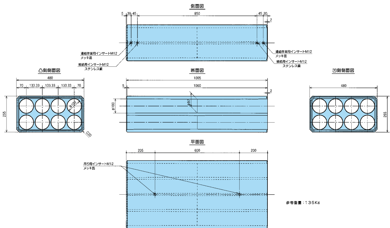
レジン多孔管直管構造図
