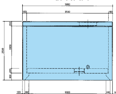
A.B視 側面図
