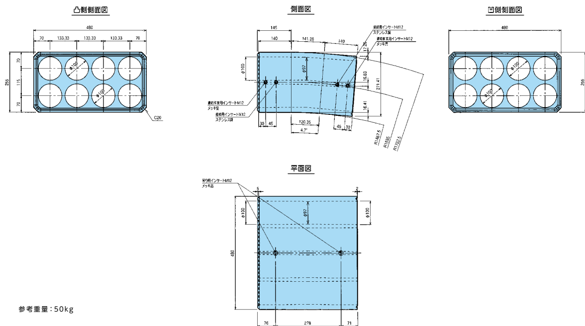
レジン多孔管垂直曲管構造図
