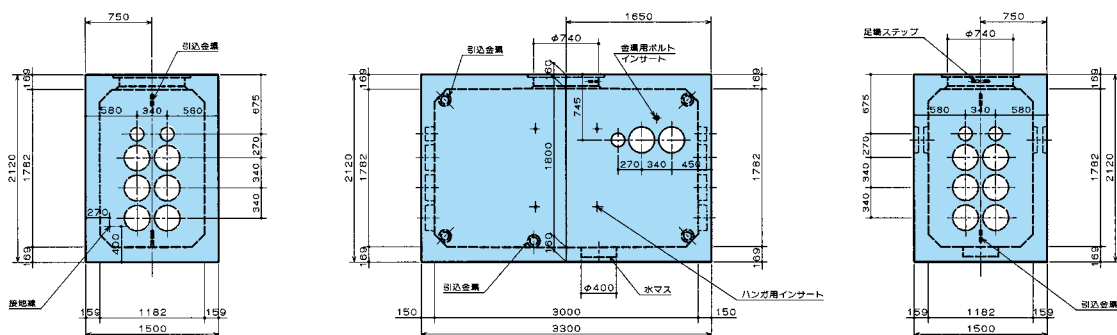
側 面 図
