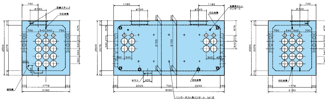
側 面 図
