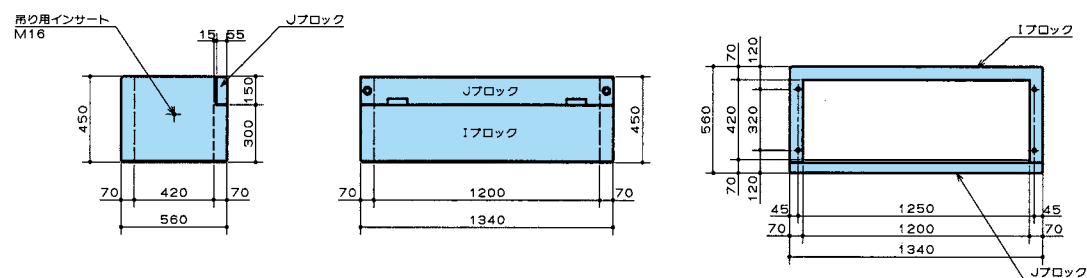
■ ハンドホールⅣ形構造図 (SWT)
