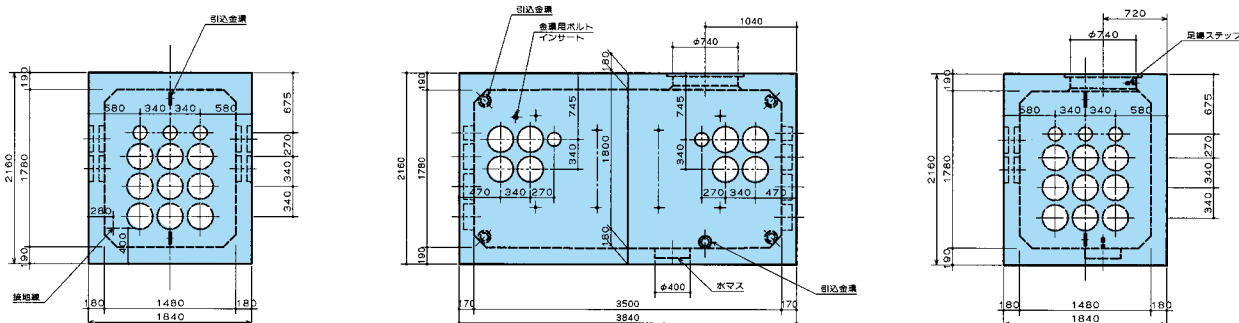
側 面 図
