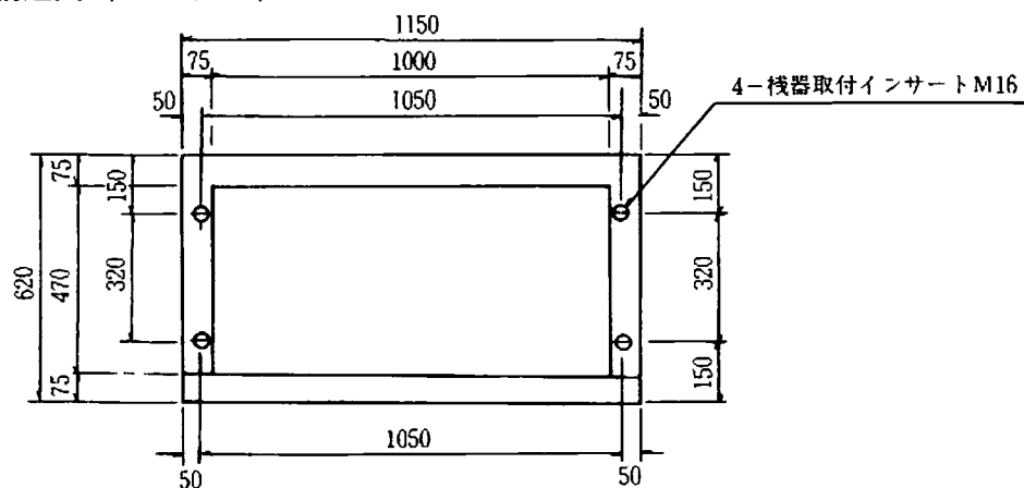
■ハンドホールⅡ形構造図（SWH、TR）
