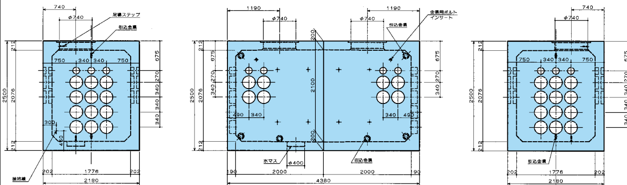
側 面 図
