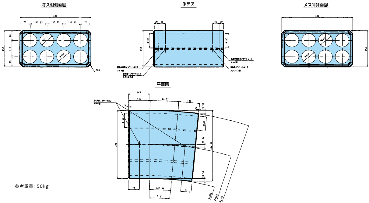
レジン多孔管水平曲管構造図
