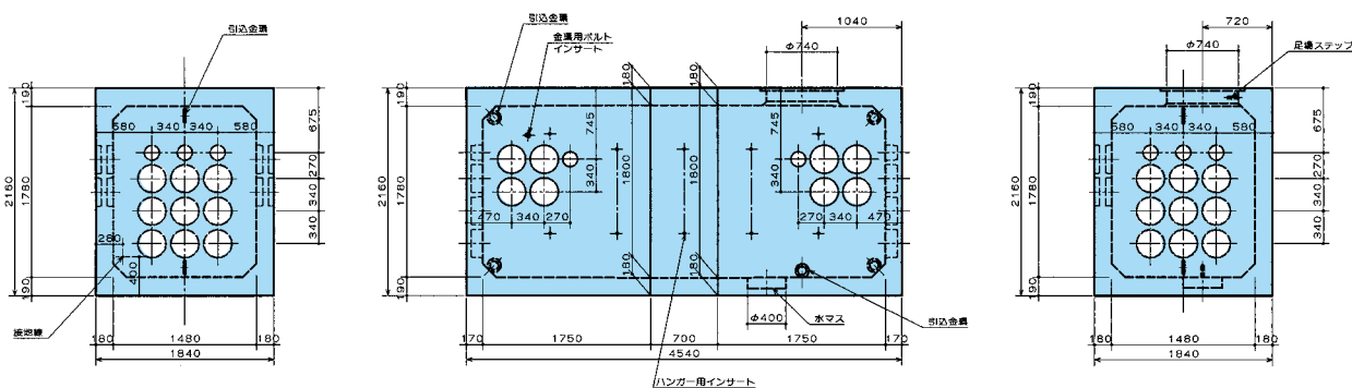
側 面 図
